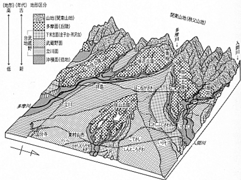
図 1-11 武蔵野台地西部の模式鳥瞰図
