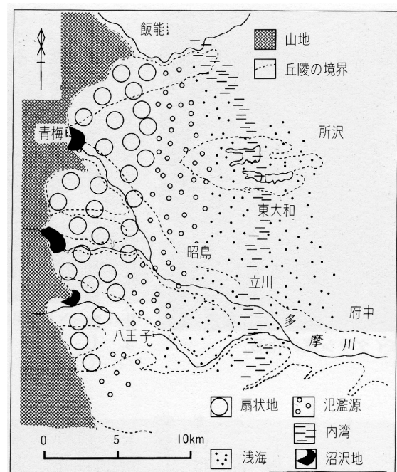
図8 関東平野西部の昔の様子 (50～200万年前)
