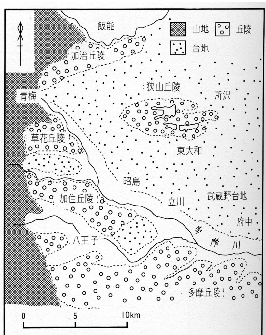
図1 関東平野西部の地形
