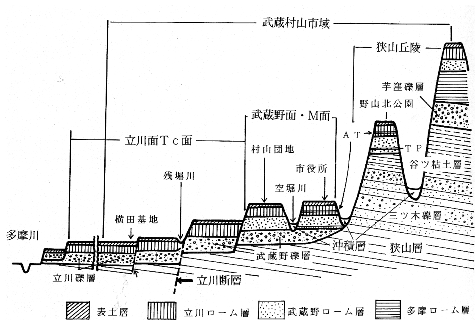
図I-3 武蔵村山市の地形断面模式図
