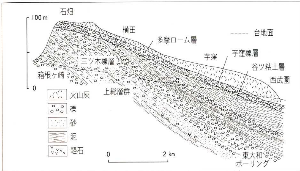
図5 狭山丘陵及び地下の地質断面図
