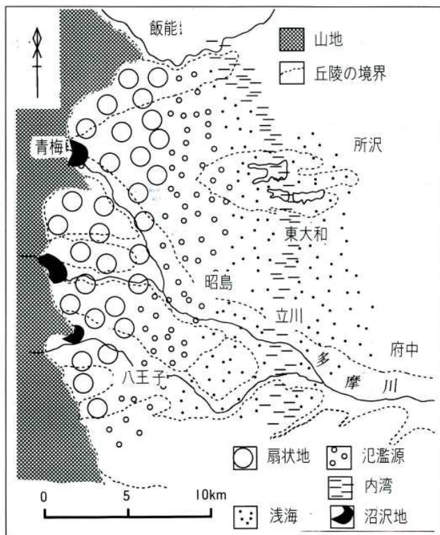
図8 関東平野西部の昔の様子 (50～200万年前)
